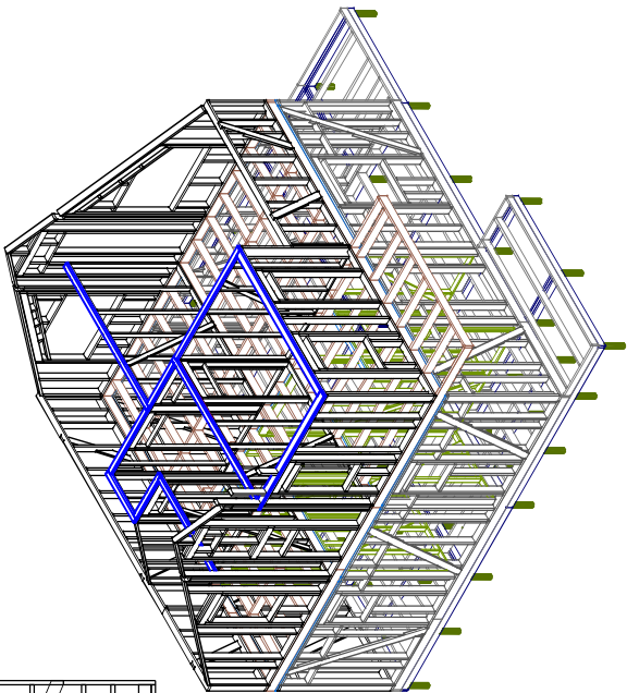
Общий вид перекрытия и рам мансарды в сборе.
