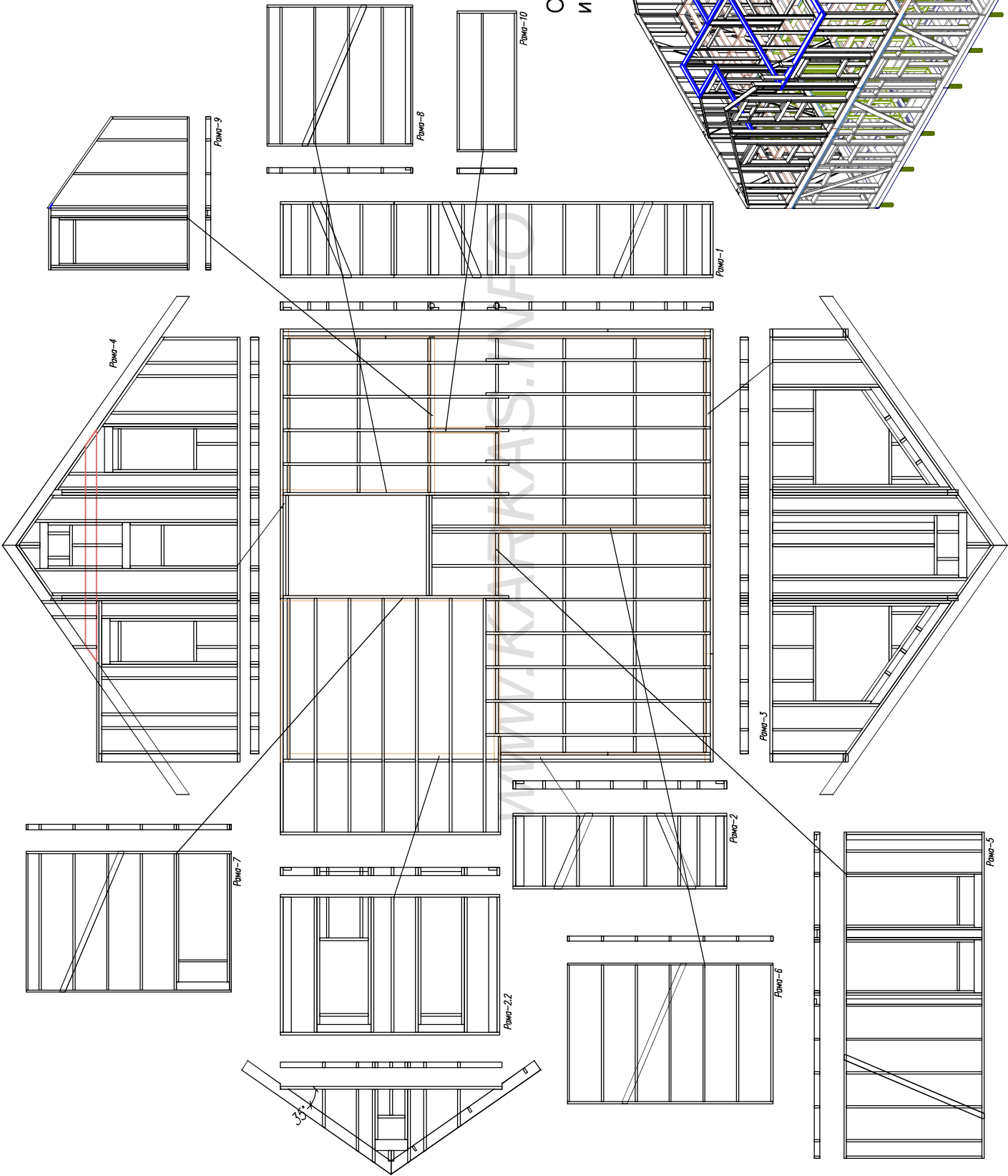
Общий вид перекрытия и рам мансарды в сборе.
